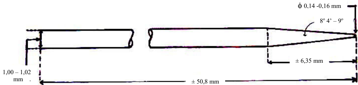
Gambar 1 - Jarum Penetrasi
